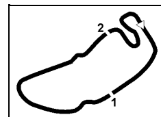
Hockenheim 6.792 m
